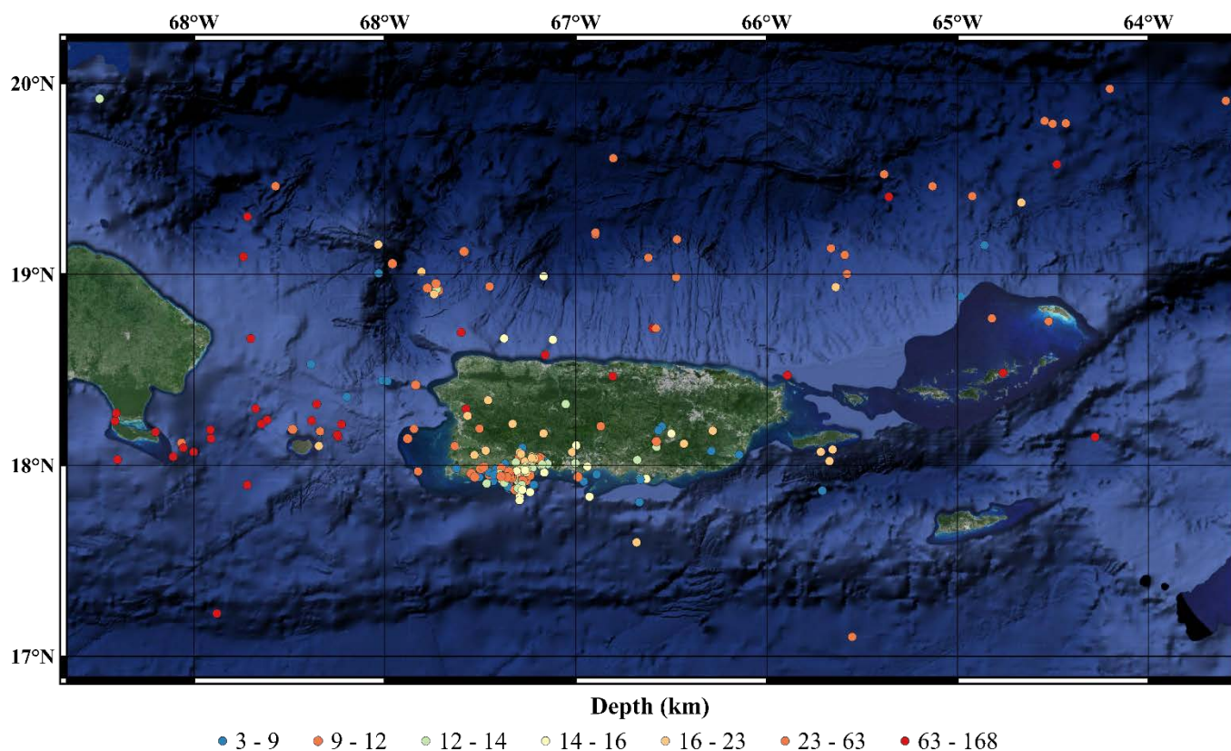
Figura 1. Mapa epicentral de los sismos localizados por la RSPR para el mes de agosto de 2025 (RSPR-UPRM).
